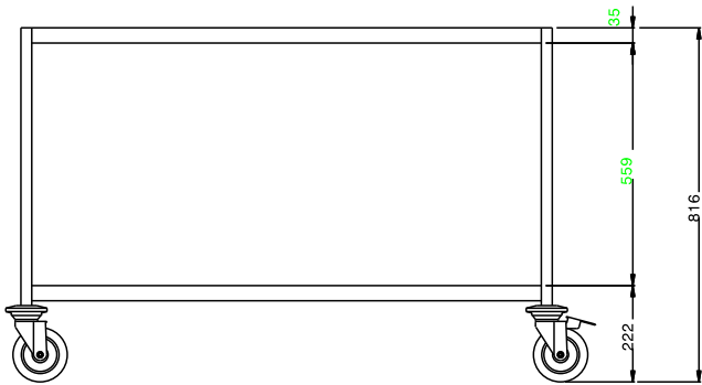
Zij aanzicht
